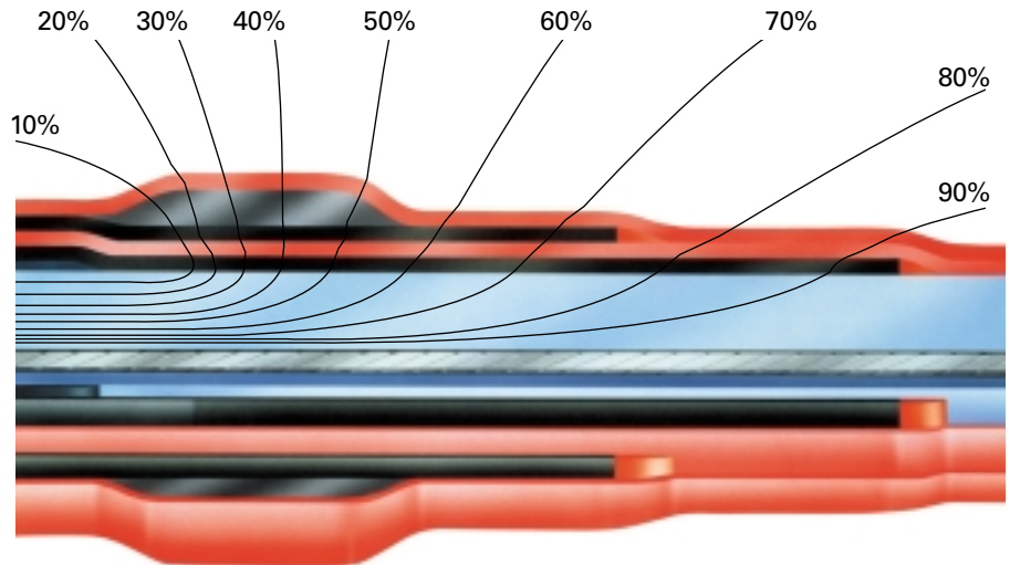
Stress plot of equipotentials
